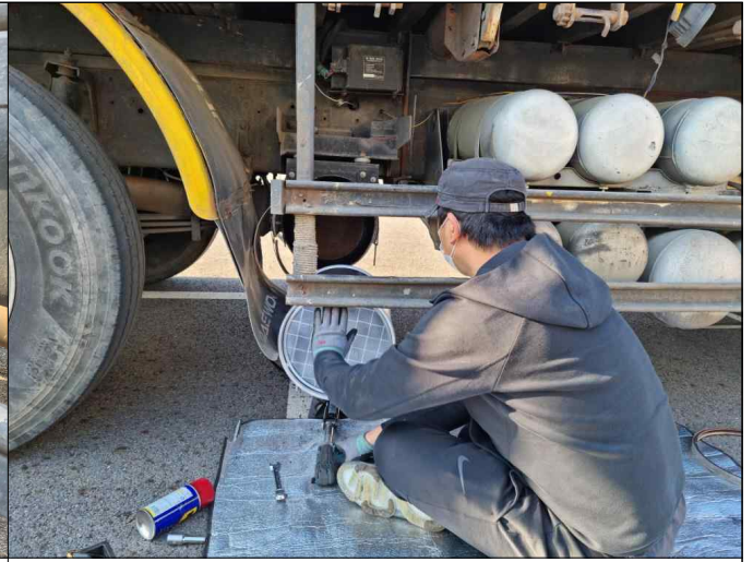
배출가스 저감장치 필터 청소
