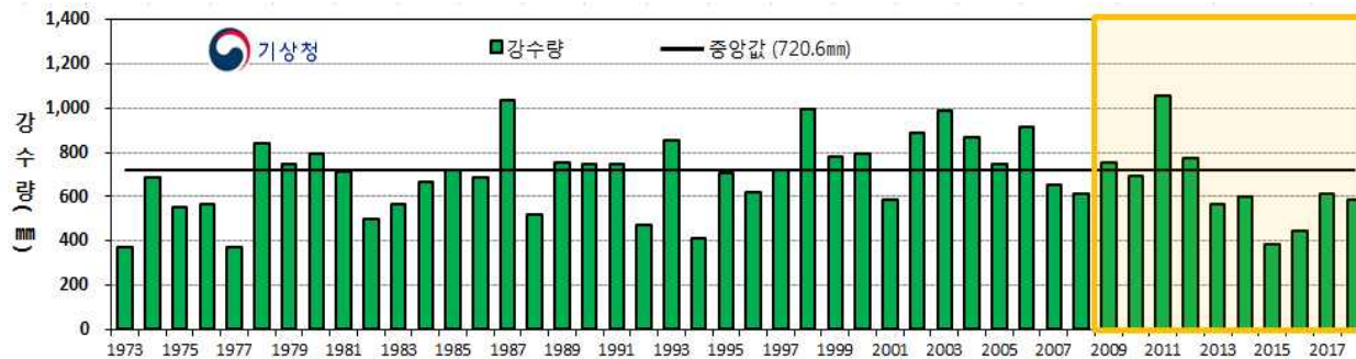
[그림 13] 연도별(1973년-2018년) 여름철 전국 평균 강수량
