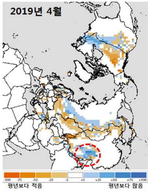
[그림 기 (왼쪽) 월별 눈 덮임 편차(4월)와 (오른쪽) 티베트 눈 덮임 편차 시계열(2018.5.18~2019.5.18)]
