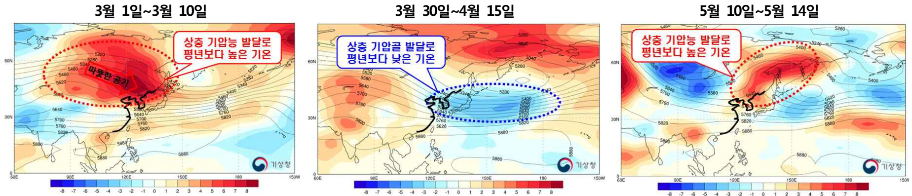
[그림 2] 500hPa(약 5.5km 상공) 지위고도(실선)와 850hPa(약 1.5km 상공) 기온 편차(채색) ※ 빨강/파랑 채색: 평년보다 높/낮은 기온
