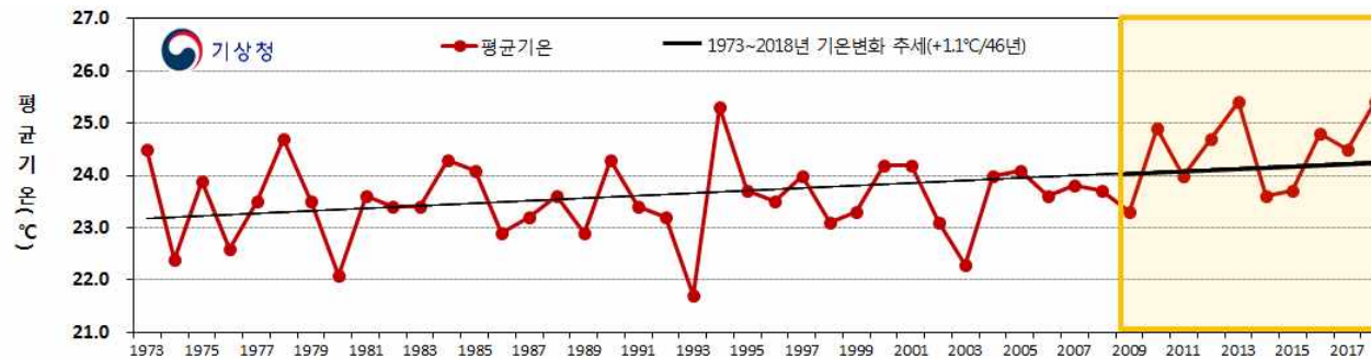
[그림 12] 연도별(1973년-2018년) 여름철 전국 평균기온
