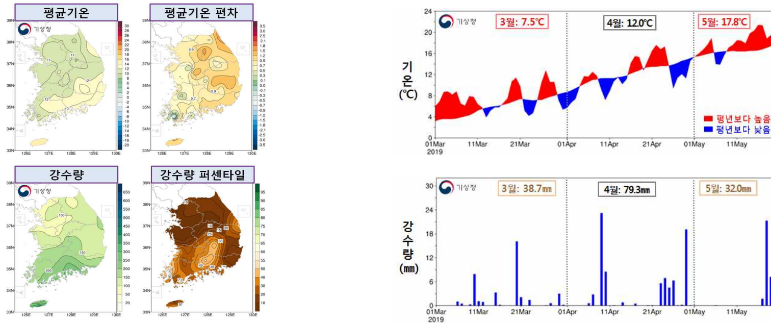
[그림 1] (위) 평균기온과 편차(°C) 분포도 및 일변화 시계열과 (아래) 강수량(mm)과 강수량 퍼센타일 분포도 및 일변화 시계열(2019.3.1~5.20.)
