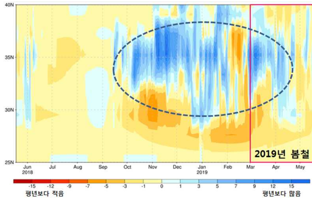
[그림 기 (왼쪽) 월별 눈 덮임 편차(4월)와 (오른쪽) 티베트 눈 덮임 편차 시계열(2018.5.18~2019.5.18)]
