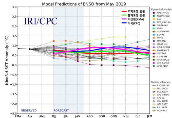
[그림 5] (왼쪽) 엘니뇨·라니냐 감시구역의 최근(5.12~5.18.) 해수면온도 편차(OISSTv2 2) )와 (오른쪽) 세계 각국의 엘니뇨·라니냐 예측 결과(출처: IRI 3) )
