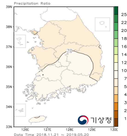
[그림 4] 최근 6개월 누적 강수량(mm)과 강수량 평년비(%) 분포도(2018.11.21~2019.5.20)
