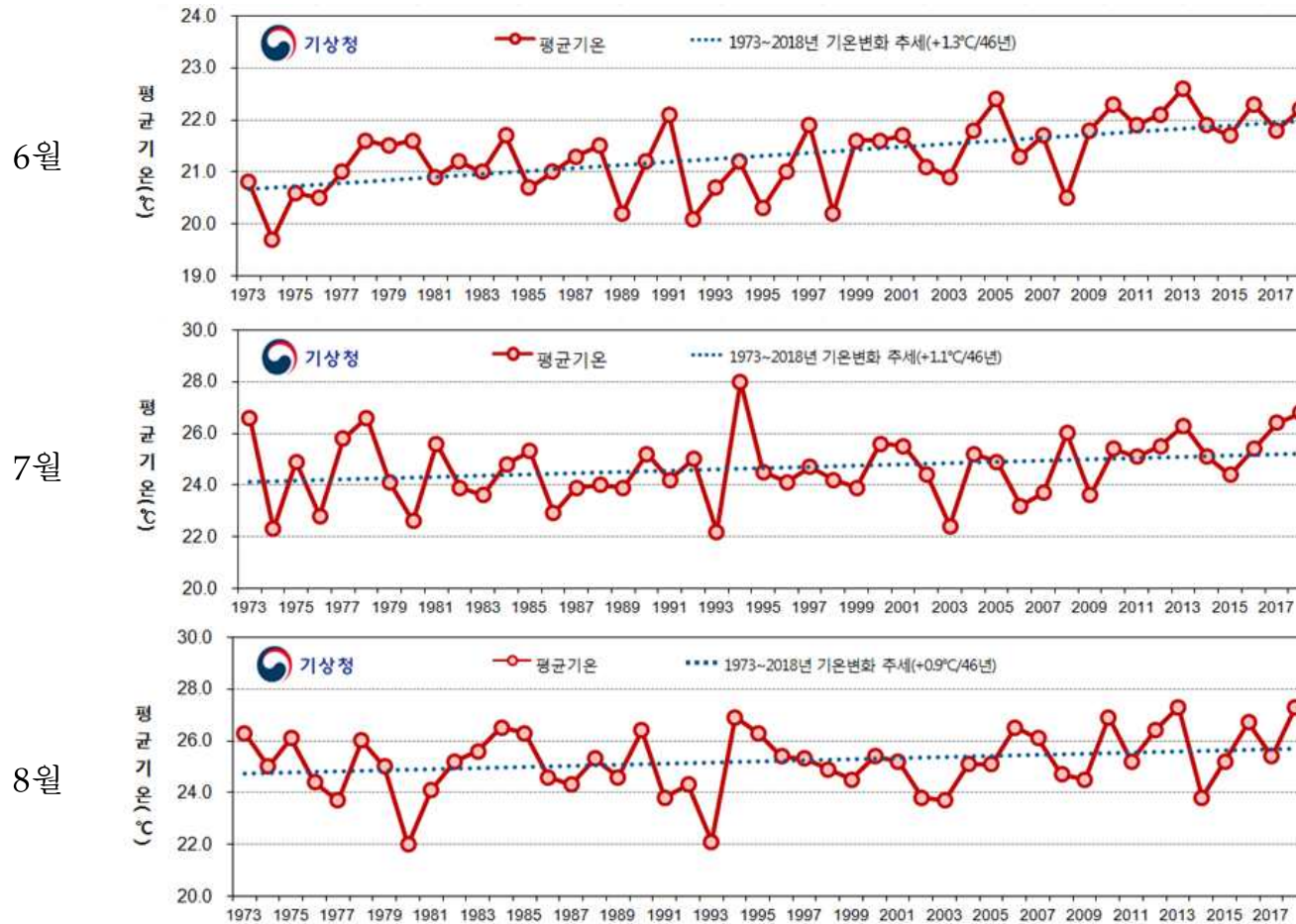
[그림 9] 연도별(1973년-2018년) 전국 월 평균기온 경향
