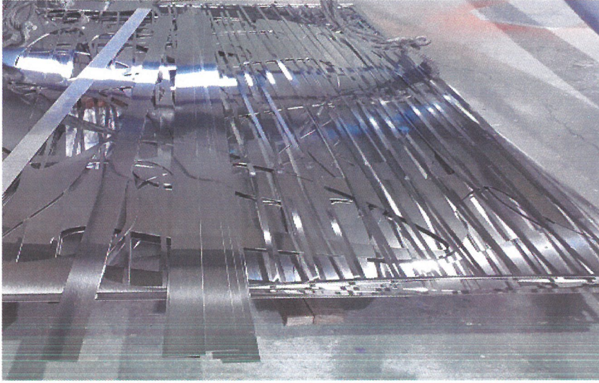
1. 상록수 파빌리온 기둥에 들어가는 레이저타공판
