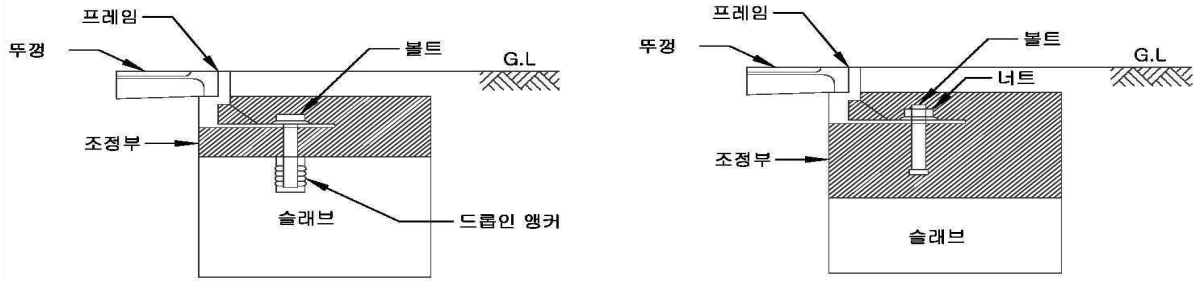
[그림5.1] 철개고정장치 설치 예시
