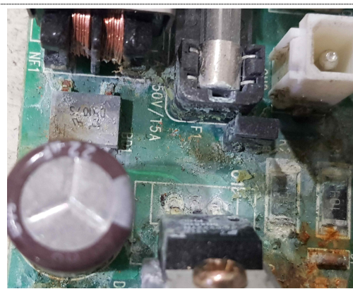
PCB 기판 탄화
