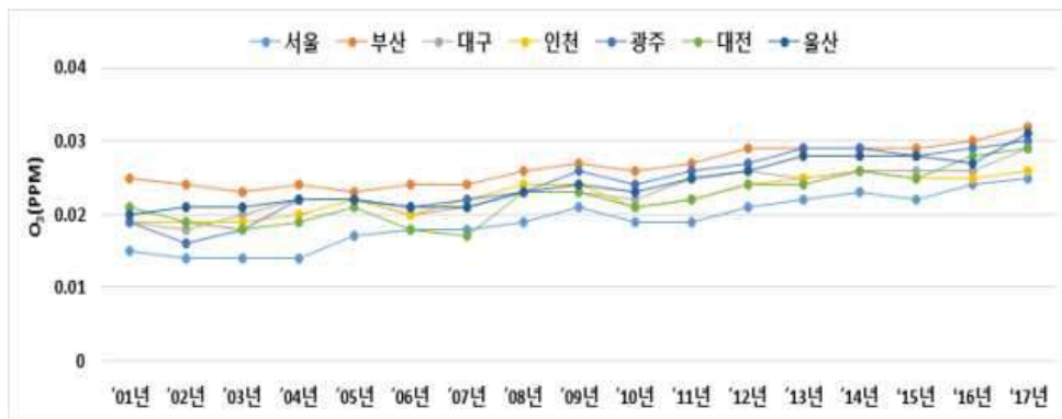
<'01~'17년 특광역시 연평균 오존 농도>
