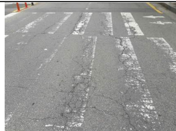
8. 횡단보도 세로방향 균열
