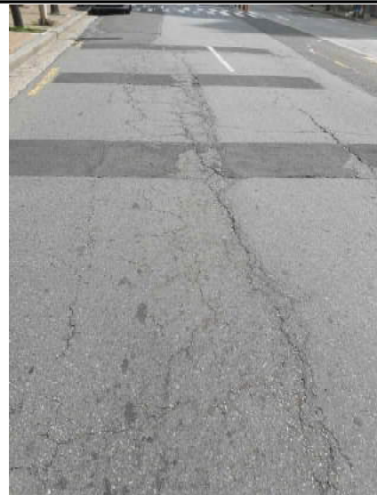
6. 침하 및 균열발생, 미끄럼방지 포장 파손
