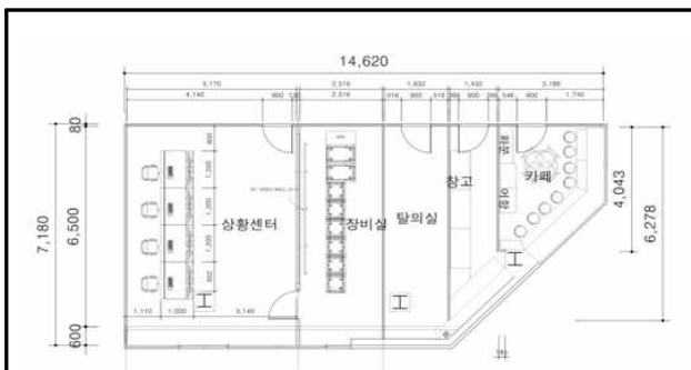
상황센터 평면도
