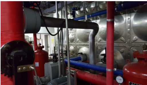
소방 펌프 성능시험배관 교체 전
