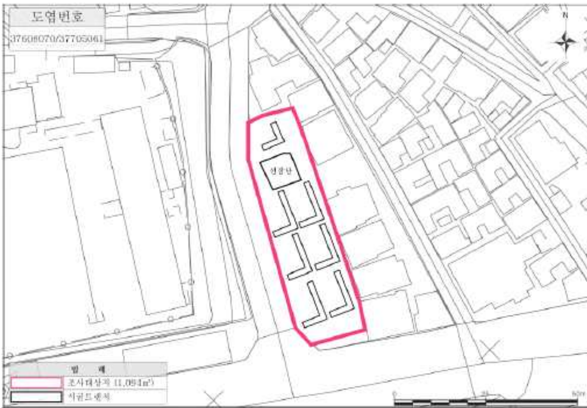
【도면 1】 트렌치 배치도(1/1000)
