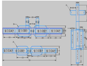
<도면 설계>
