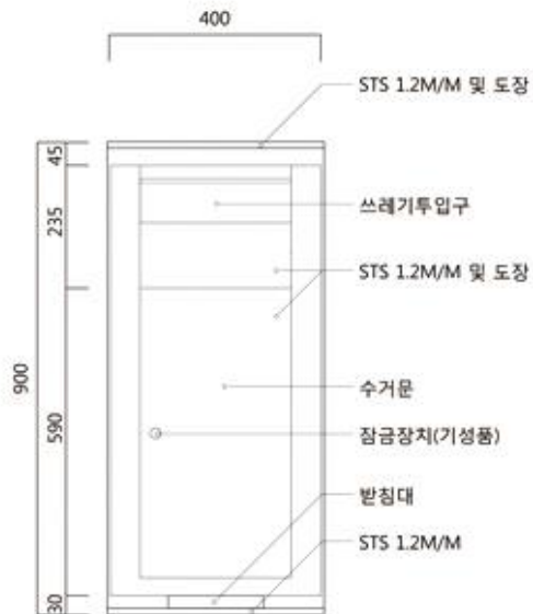
[정면도]
