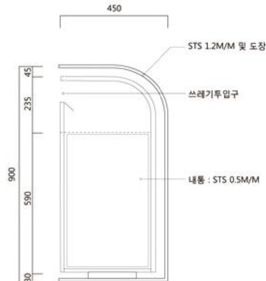
[측면도]
